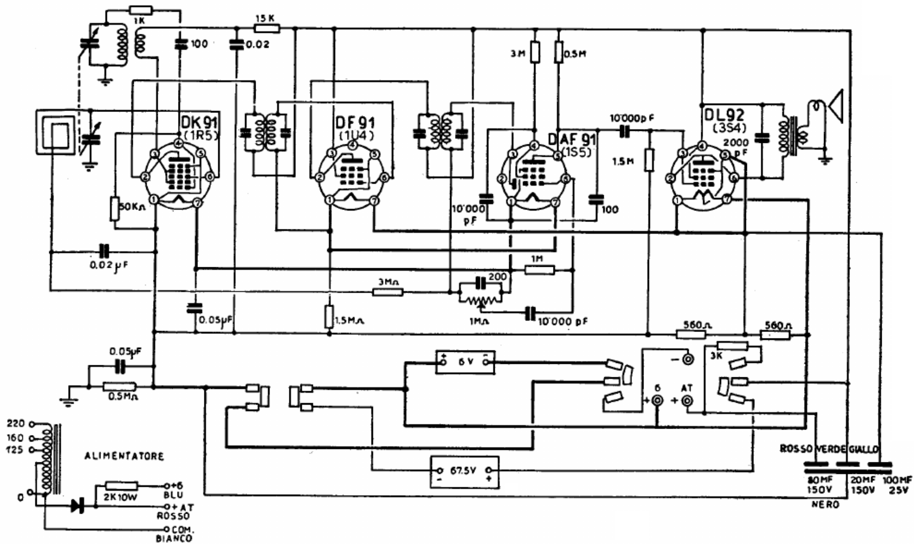
FARA RADIO - Mod. MICKEY - Portatile a pile, con funzionamento automatico ad apertura del coperchio. Alimentabile dalla rete-luce con adattatore esterno inseribile con spinetta tripolare. Dimensioni dell'apparecchio 21×10×6 cm.
